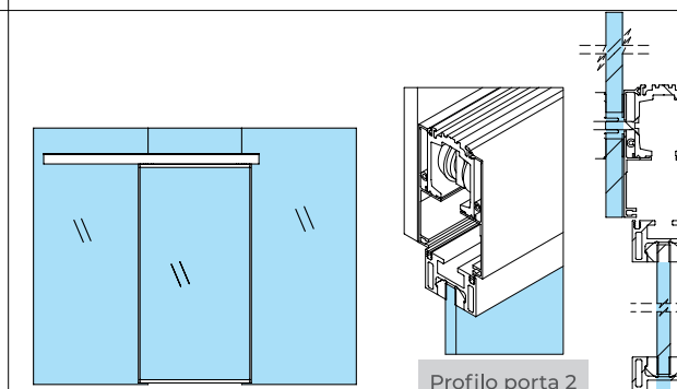
Door profile 2 | Perfil puerta 2
