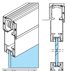
Door profile 1 | Perfil puerta 1
