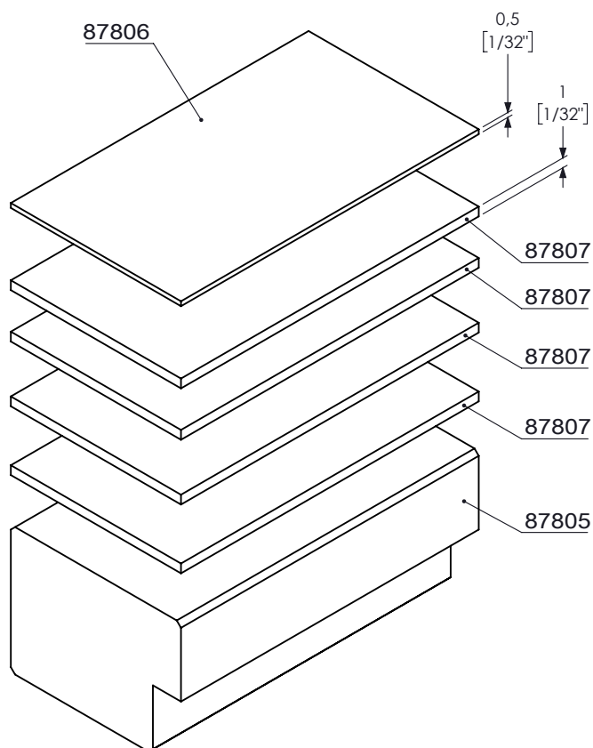
Kit distanziali vetro Kit glass spacer Kit distancias para vidrio
