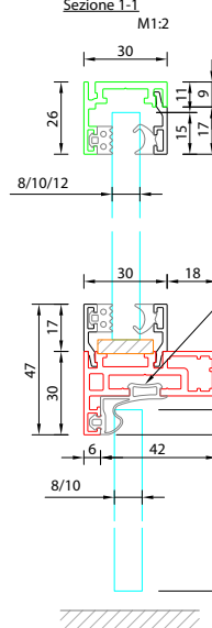
Section 1-1 Sezione 1-1
