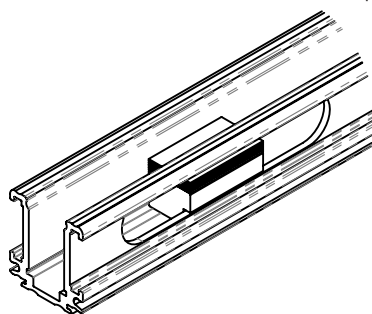
Kit distanziali vetro Kit glass spacer Kit distancias para vidrio
