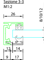
Section 3-3 Sezione 3-3
