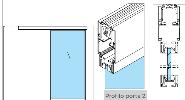
Door profile 2 | Perfil puerta 2
