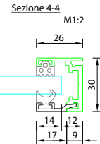
Section 4-4 Sezione 4-4
