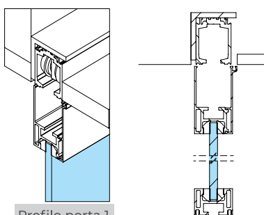
Door profile 1 | Perfil puerta 1
