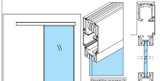
Door profile 2 | Perfil puerta 2
