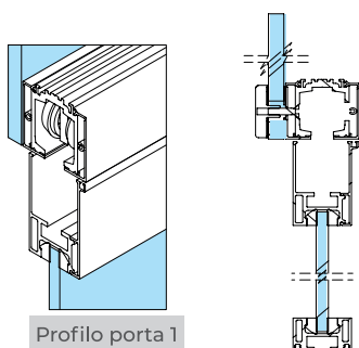
Door profile 1 | Perfil puerta 1
