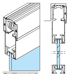
Door profile 1 | Perfil puerta 1
