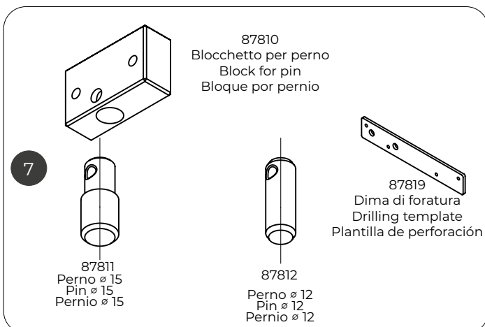
87819 Dima di foratura Drilling template Plantilla de perforación
